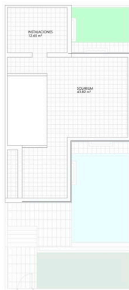
PLANTA ATICO 1 : 100
